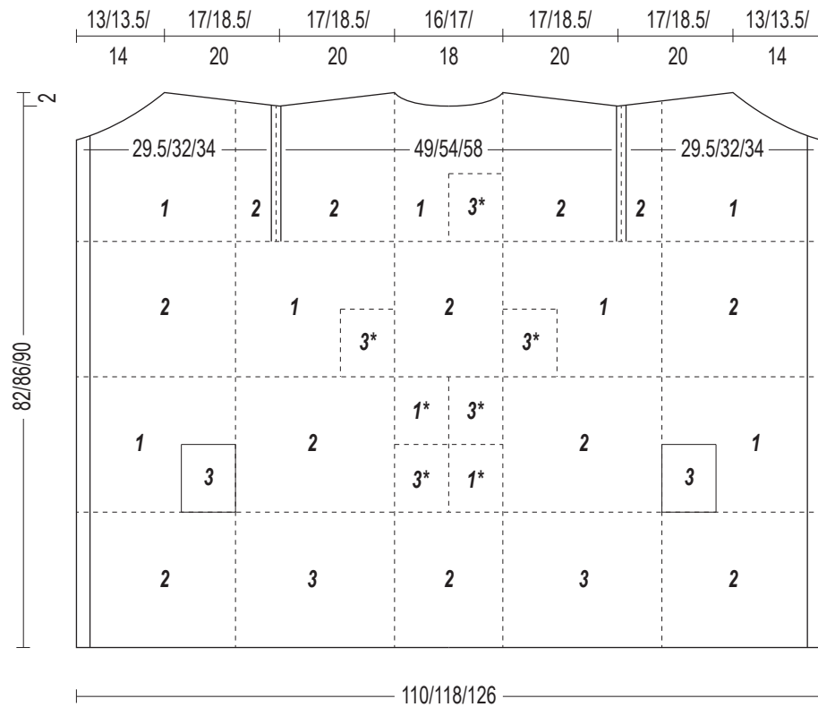
Schnittskizze 1 / pat sketches 1 / section croquis 1 / sectie schets 1
